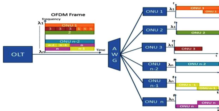
Fig. 5. OFDM/WDM-PON.
