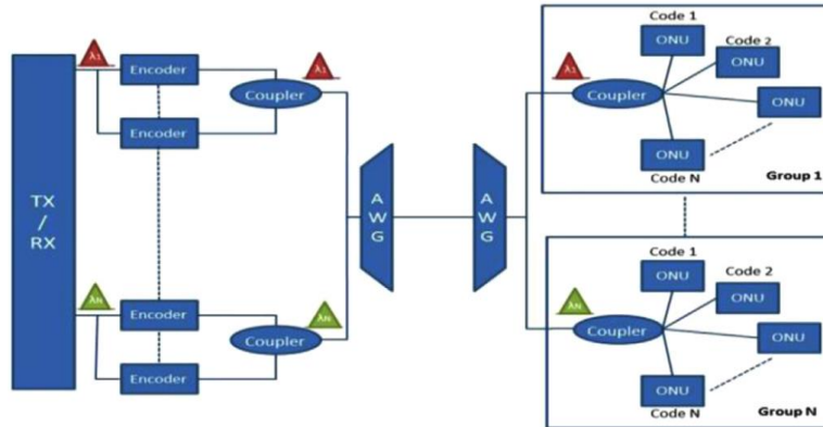
Fig. 4. OCDM/WDM-PON.
